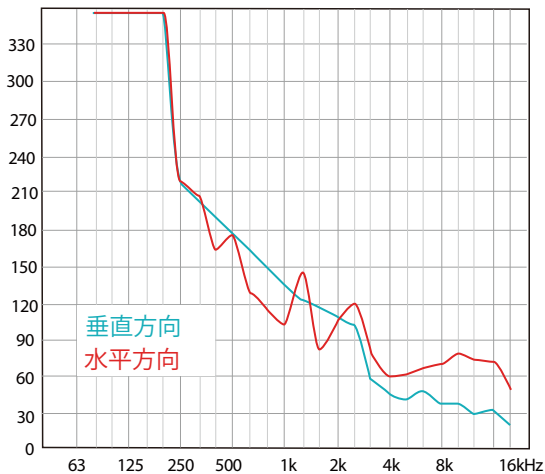
a-10 指向特性
