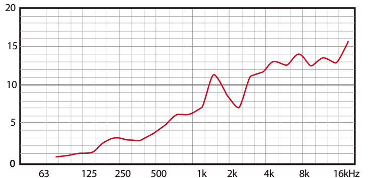
a-10 指向係数 (dB)
